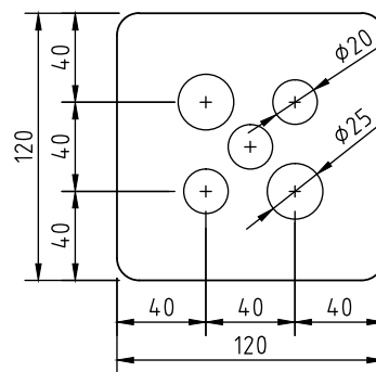
CONDUIT LOCATION BOX BASE
